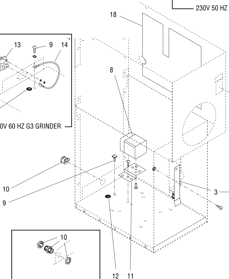
230V 50 HZ G1, G2 & G3 GRINDERS
