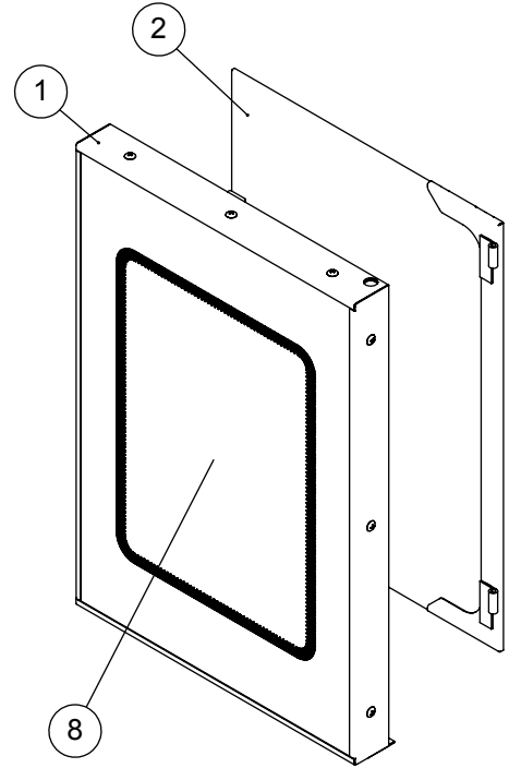
RH DOOR
