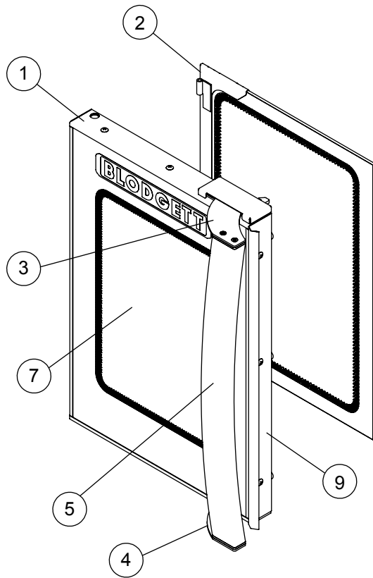
LH DOOR
